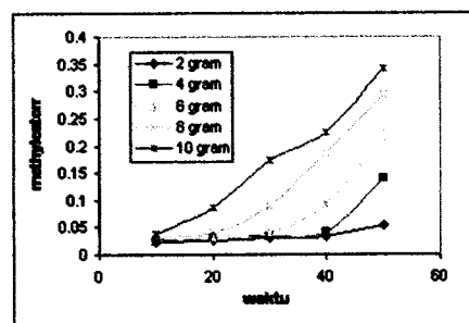
Gambar 2. Hubungan antara area percent methyl ester dengan waktu Proses pada berbagai banyaknya zeolit.
