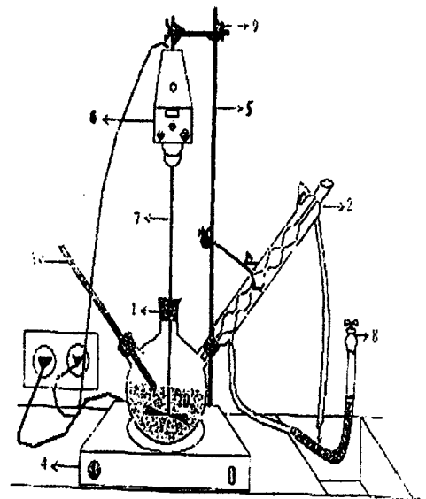
Gambar 1. Rangkaian alat
