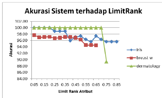
Gambar 6. Grafik pengaruh limit gain ratio terhadap akurasi.
