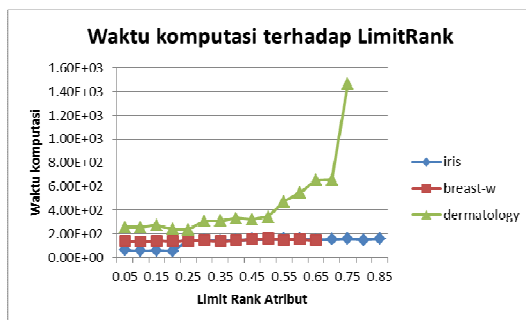
Gambar 7. Grafik pengaruh limit gain ratio terhadap waktu komputasi
