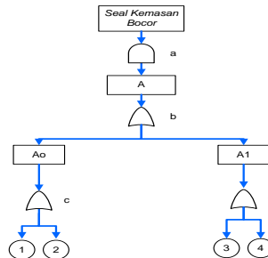
Gambar 5 Struktur Kecacatan Seal Kemasan Bocor
